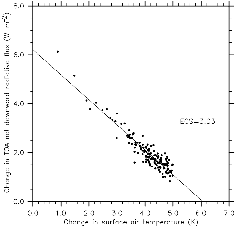
(b) BCC-CSM1.1m
