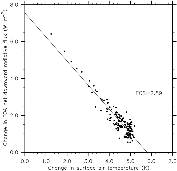
(b) BCC-CSM1.1m
